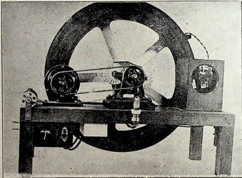
Een televisior, uit zelfvervaardigde onderdelen omgebouwd.
