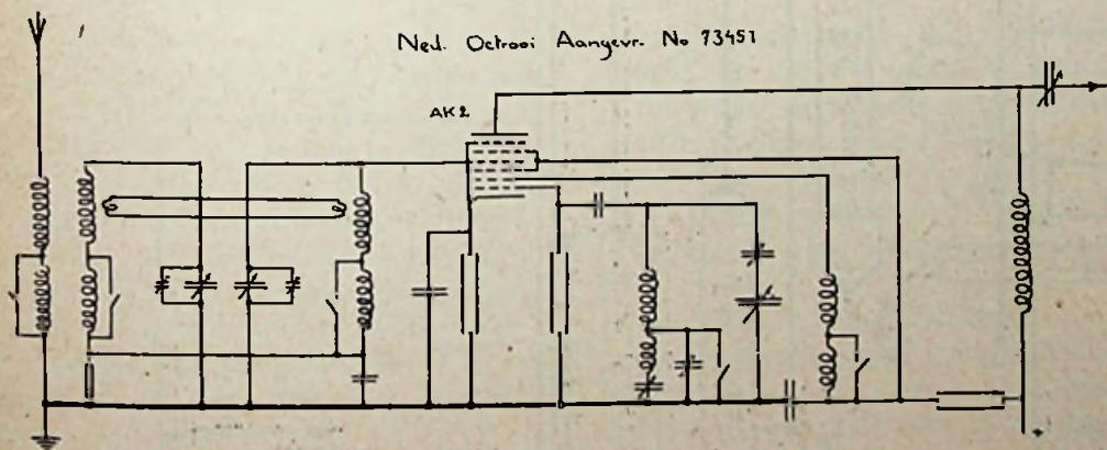
Nijkerk's Radio Super Select zonder UKG
